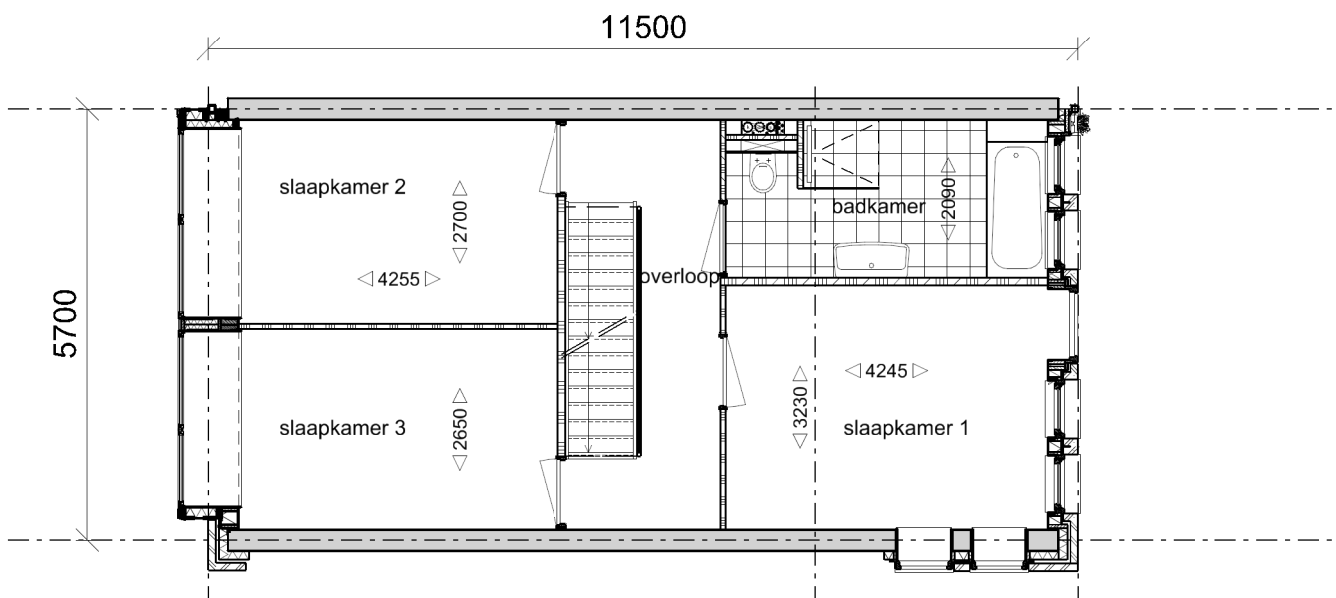
Verdieping 1
