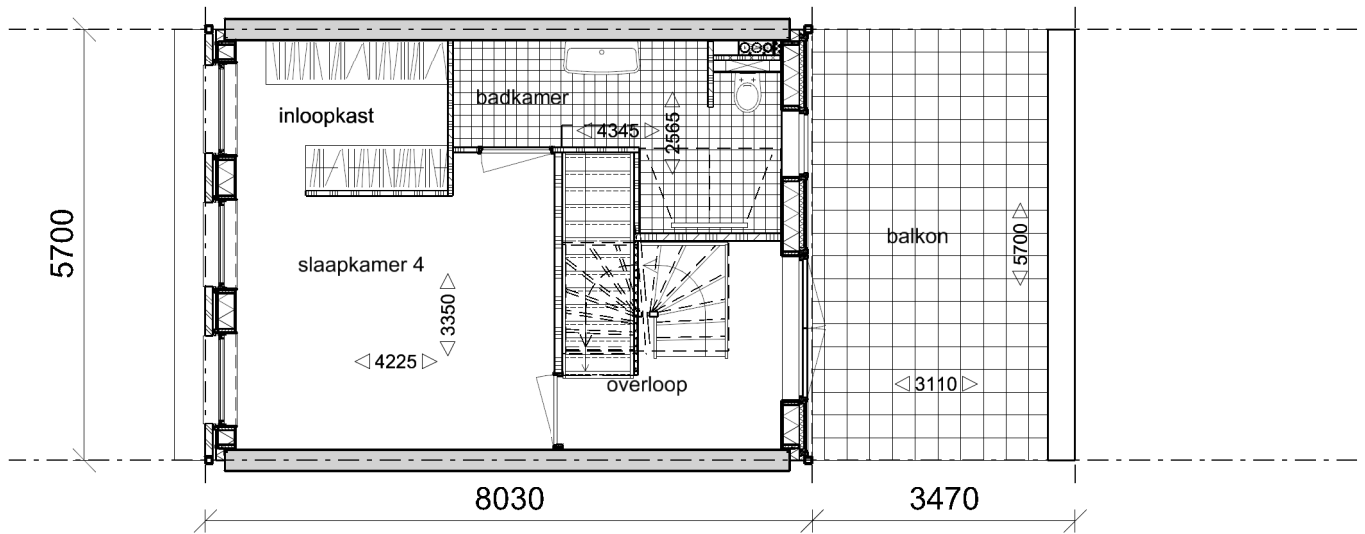
Verdieping 2
