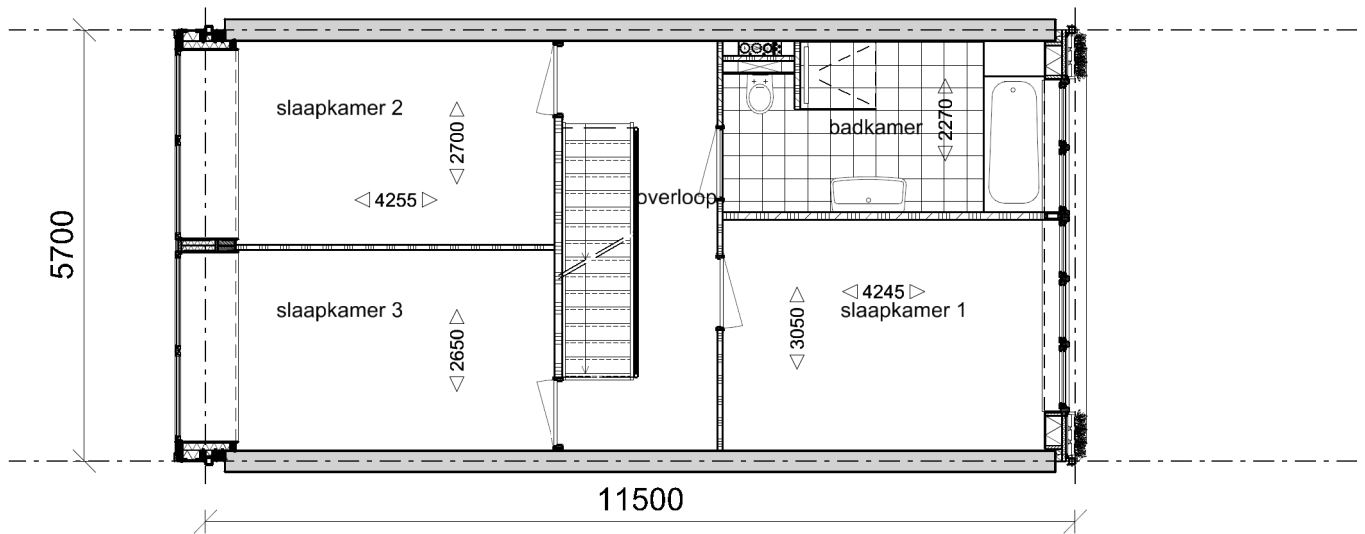
Verdieping 1
