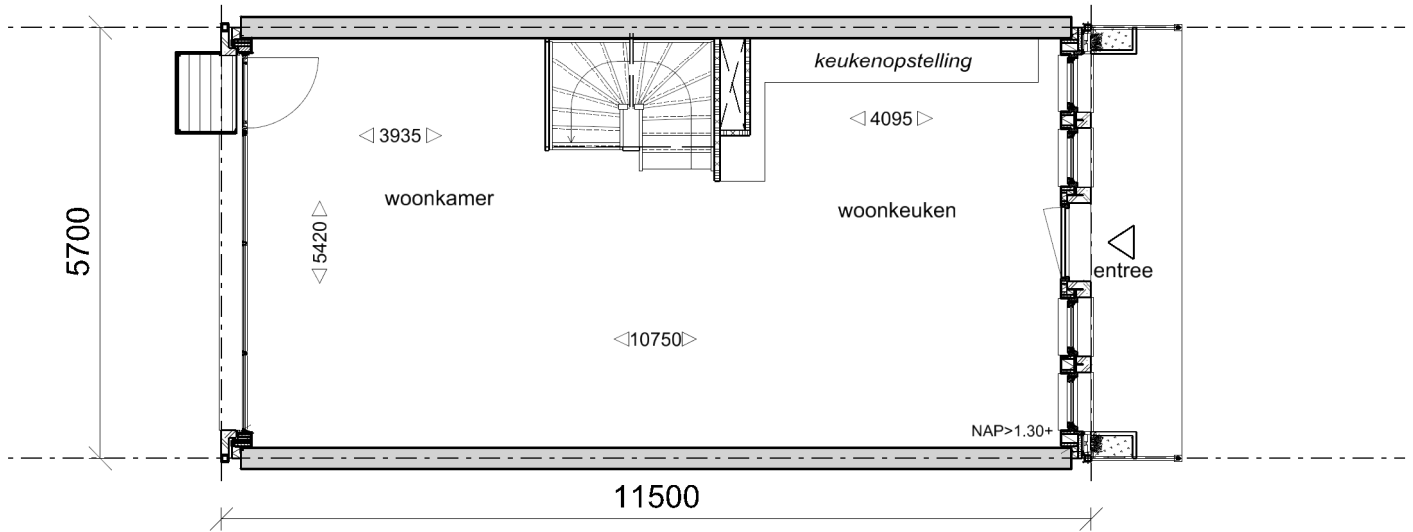
Begane grond
