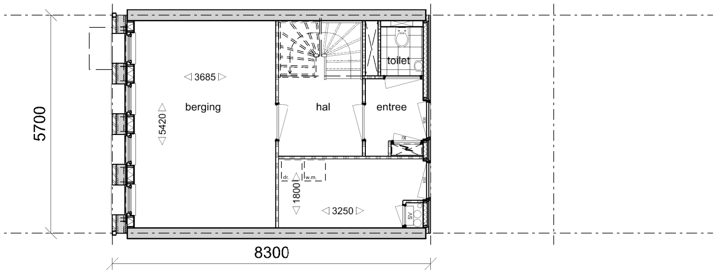
Souterrain
