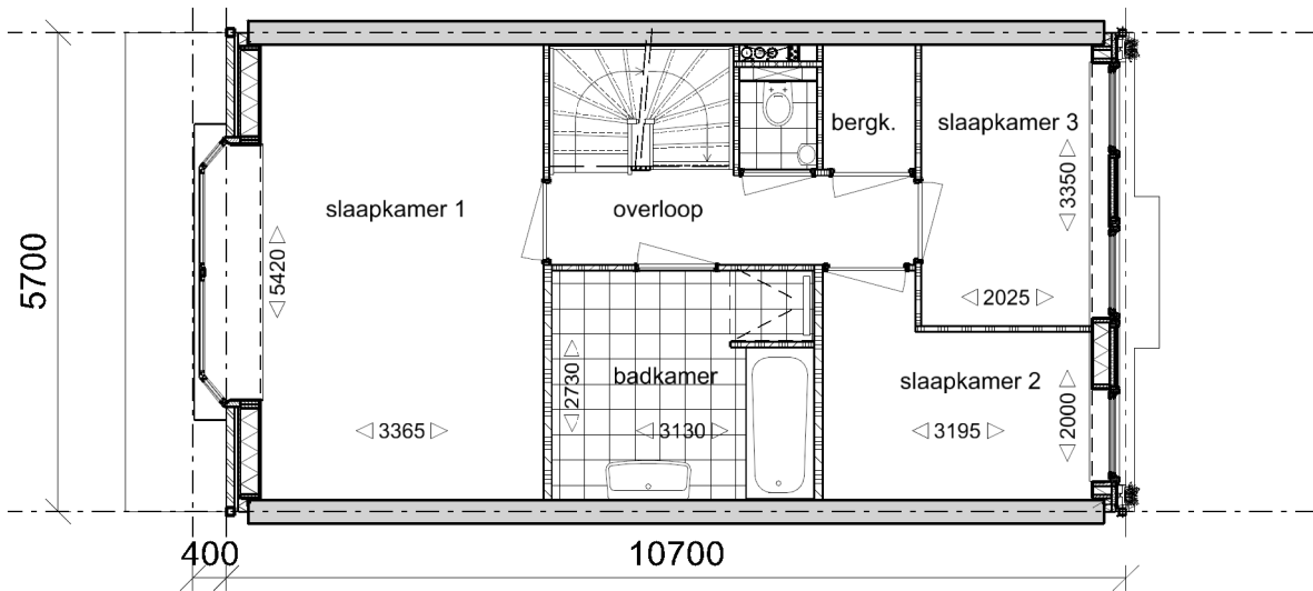
Verdieping 1
