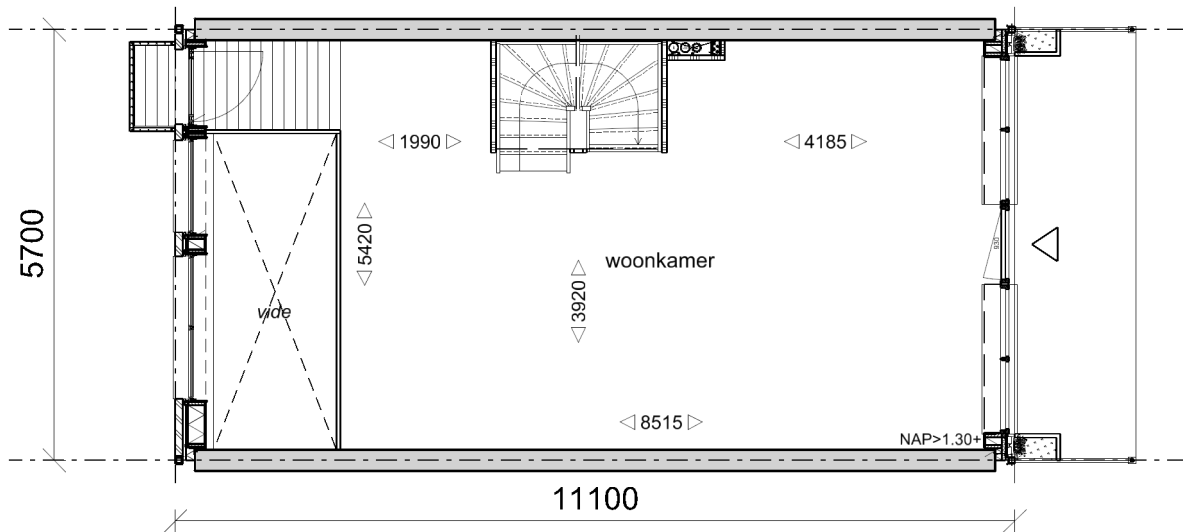
Begane grond
