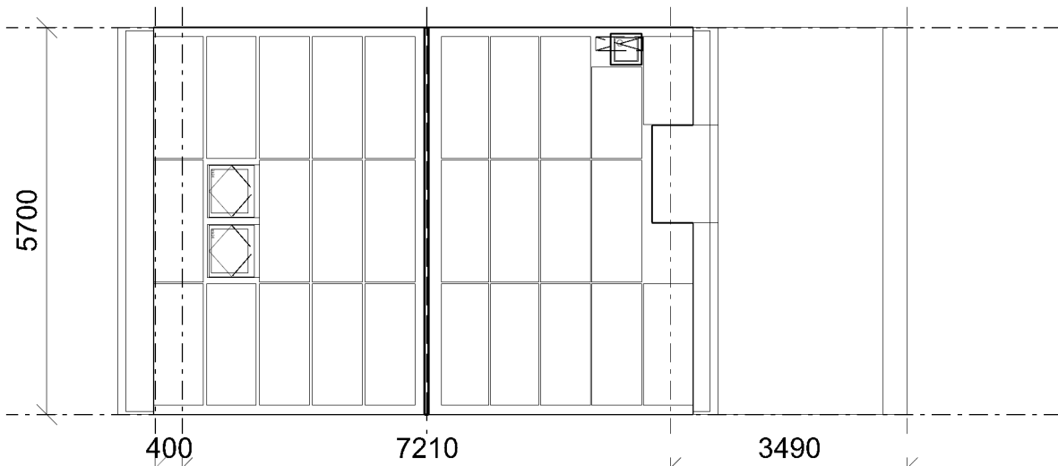
Dakaanzicht
