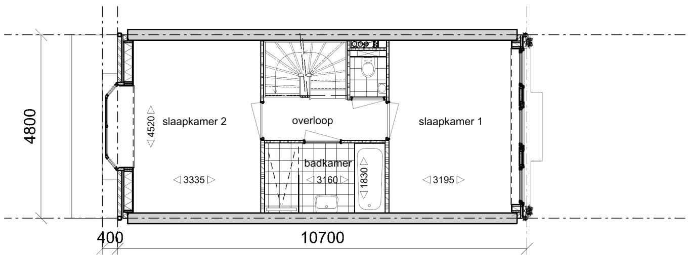
Verdieping 1
