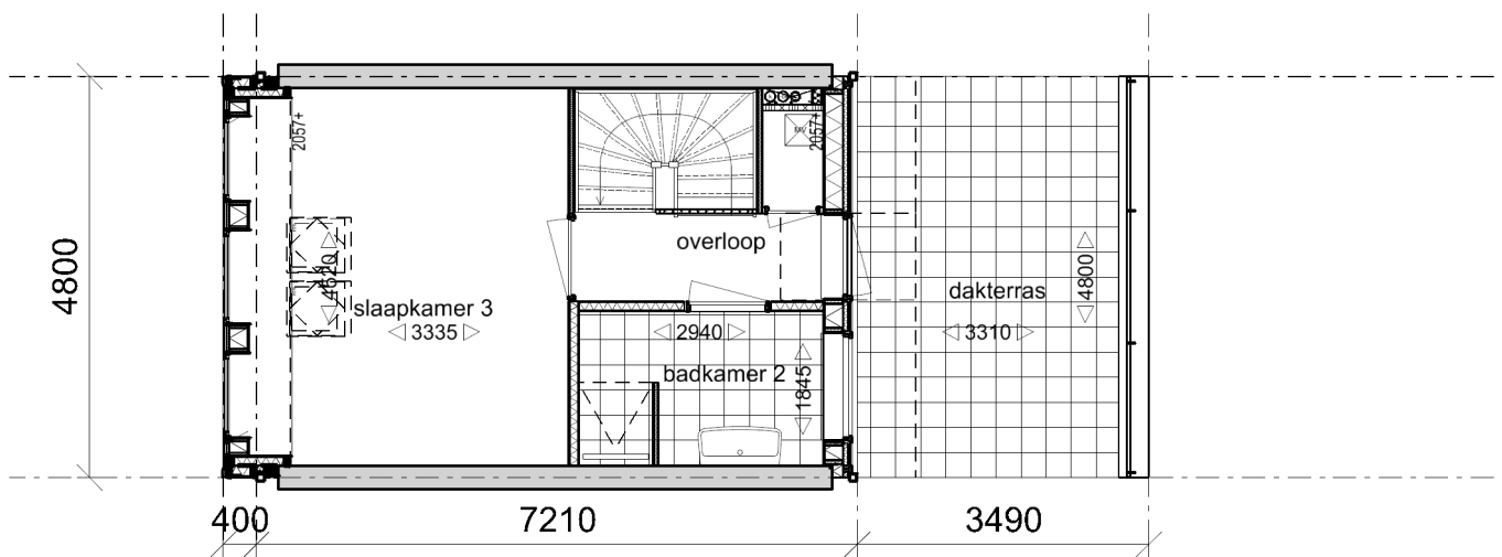
Verdieping 2
