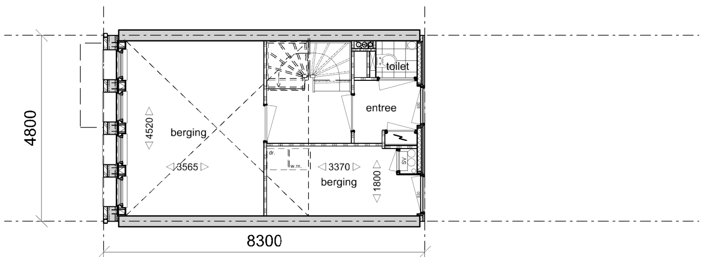
Souterrain
