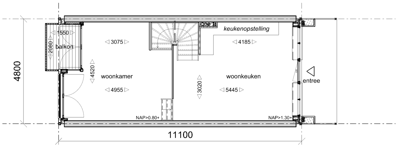
Begane grond
