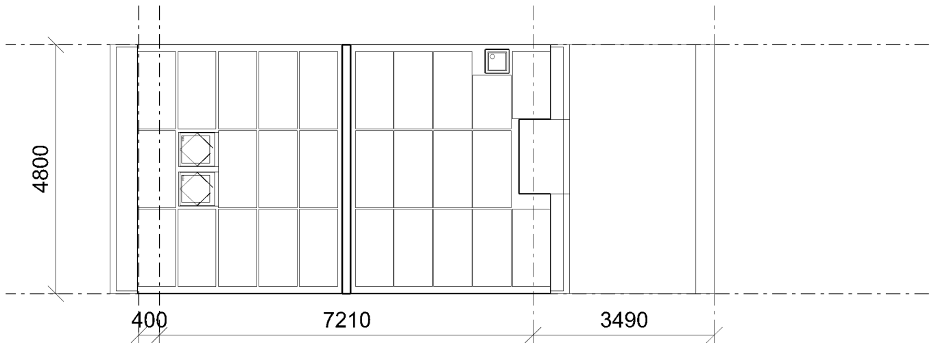
Dakaanzicht
