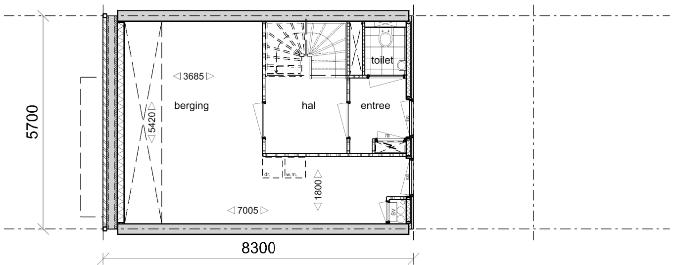
Souterrain
