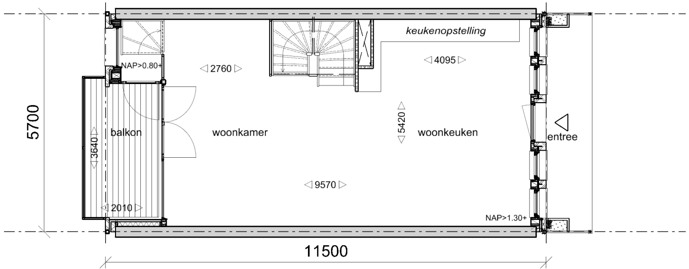
Begane grond
