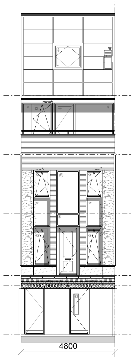
Gevel Straatzijde
