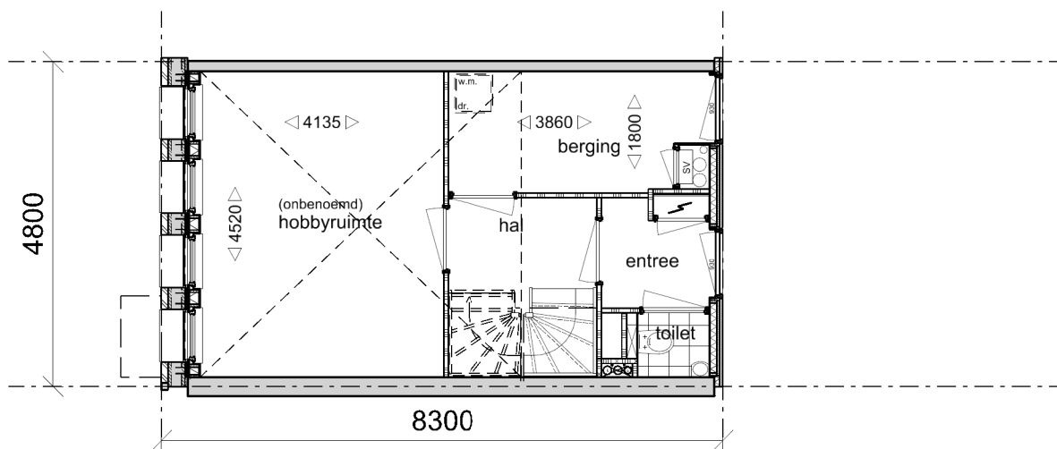
Souterrain
