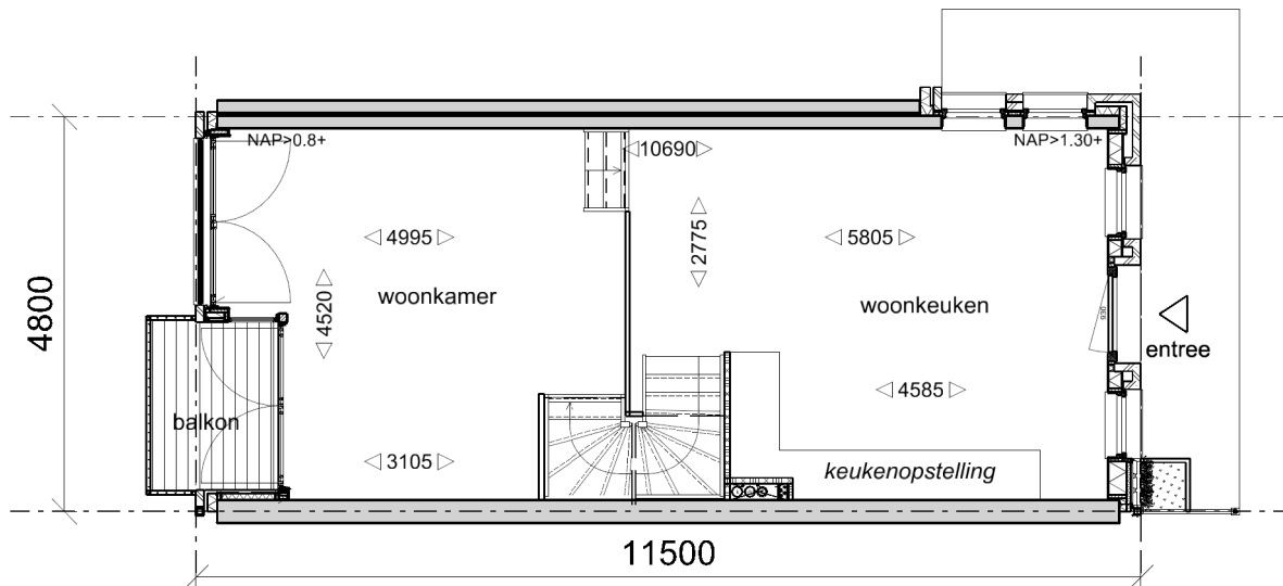
Begane grond
