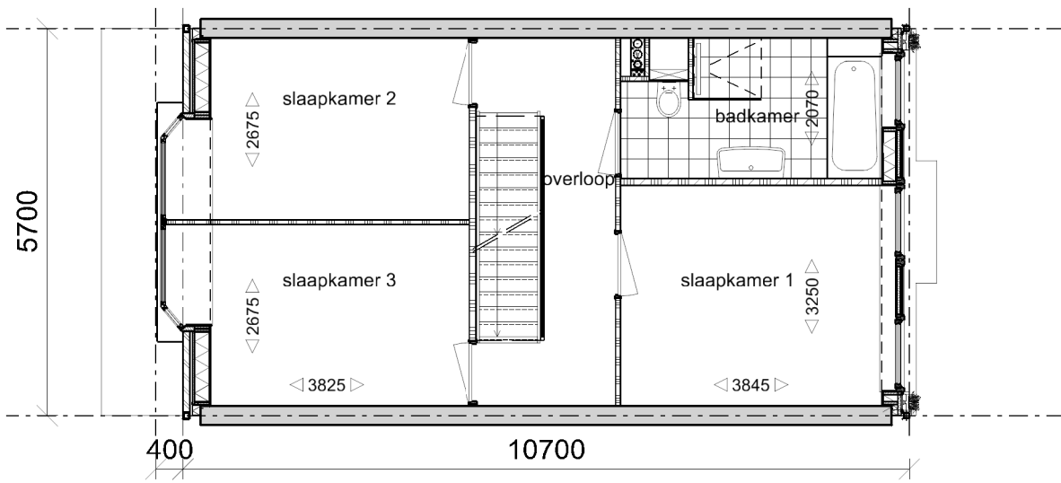
Verdieping 1
