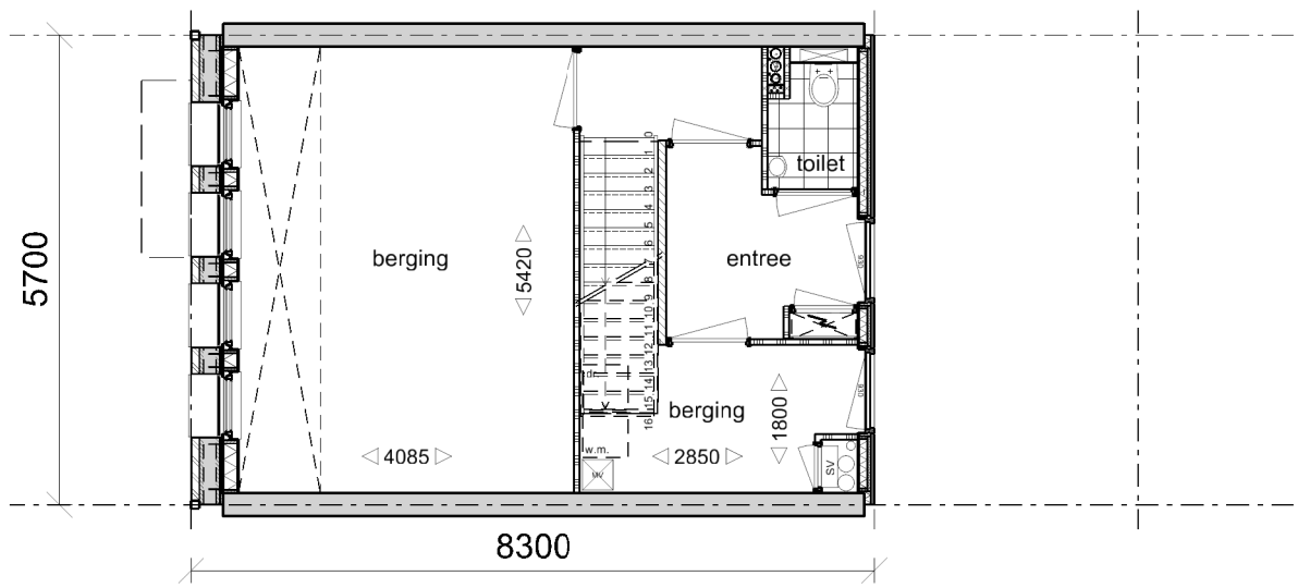
Souterrain
