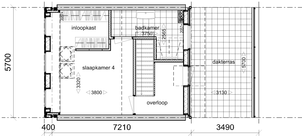
Verdieping 2
