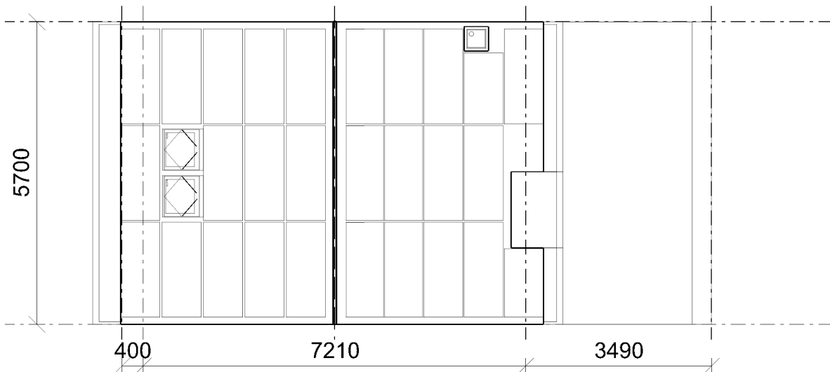
Dakaanzicht
