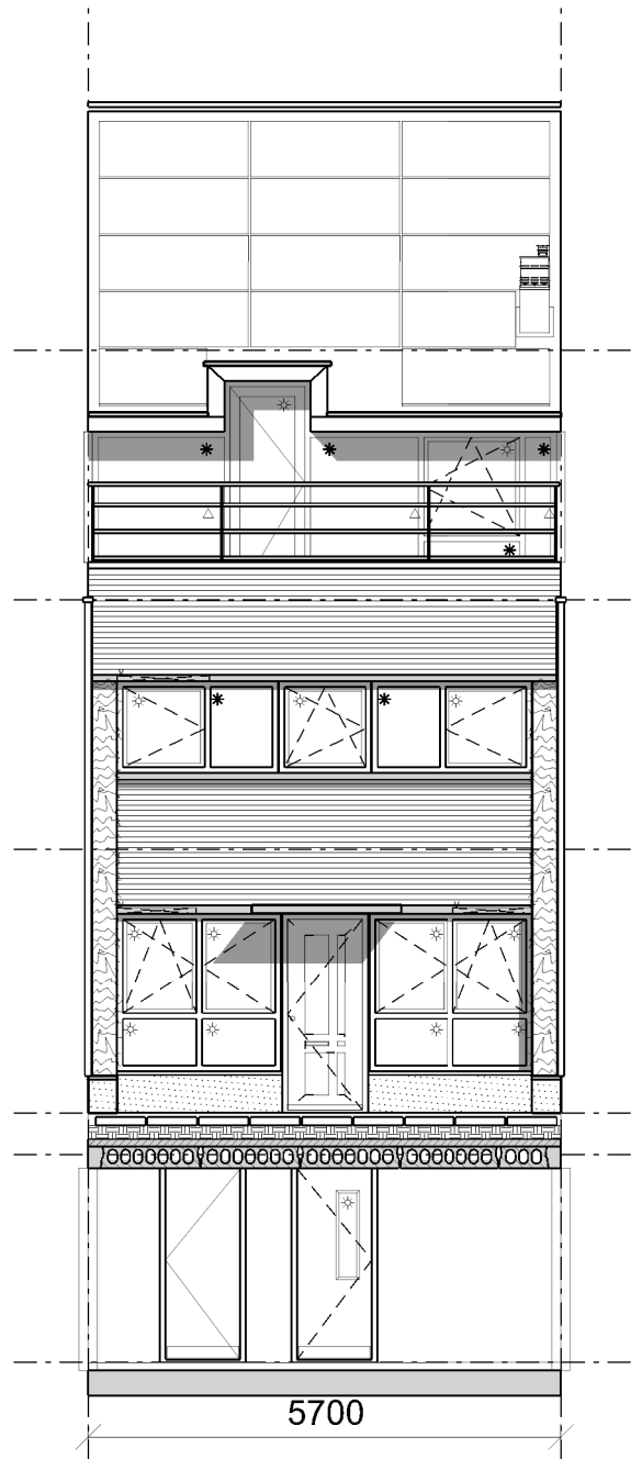
Gevel Straatzijde
