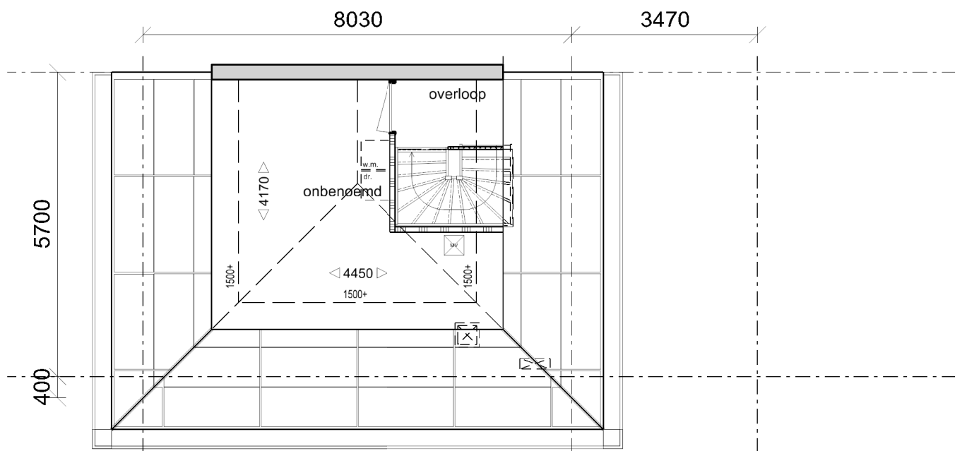
Verdieping 3
