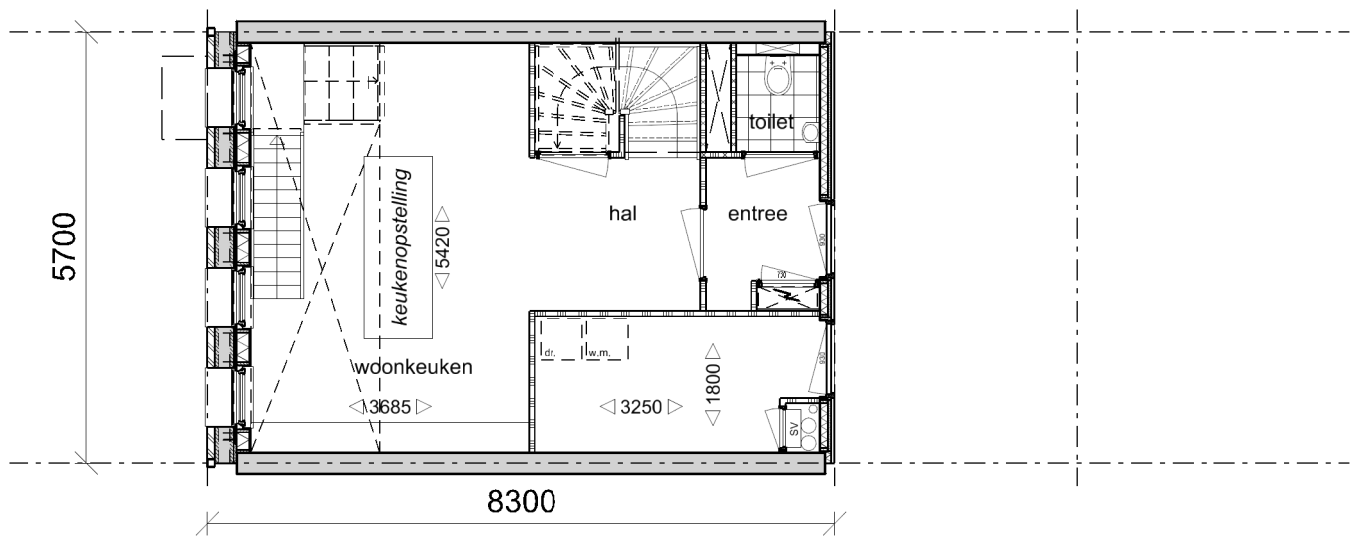
Souterrain
