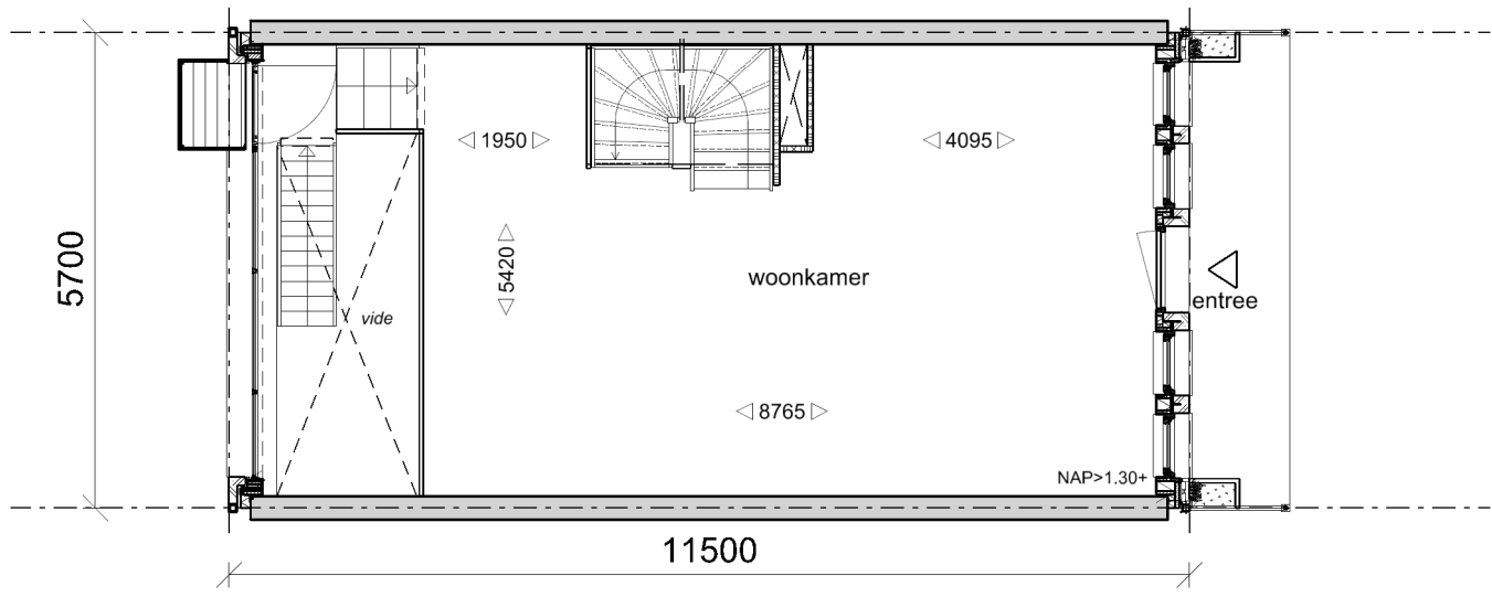
Begane grond
