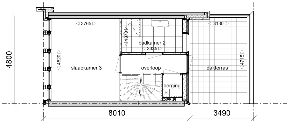
Verdieping 2
