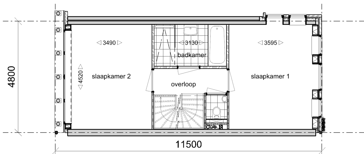
Verdieping 1
