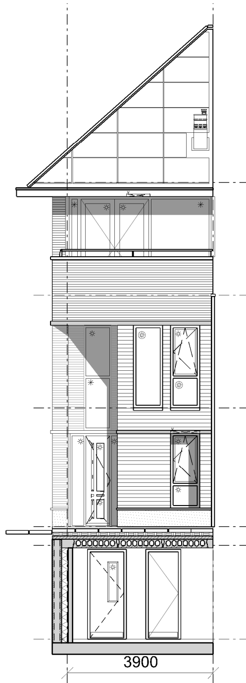
Gevel Straatzijde
