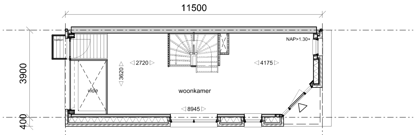
Begane grond
