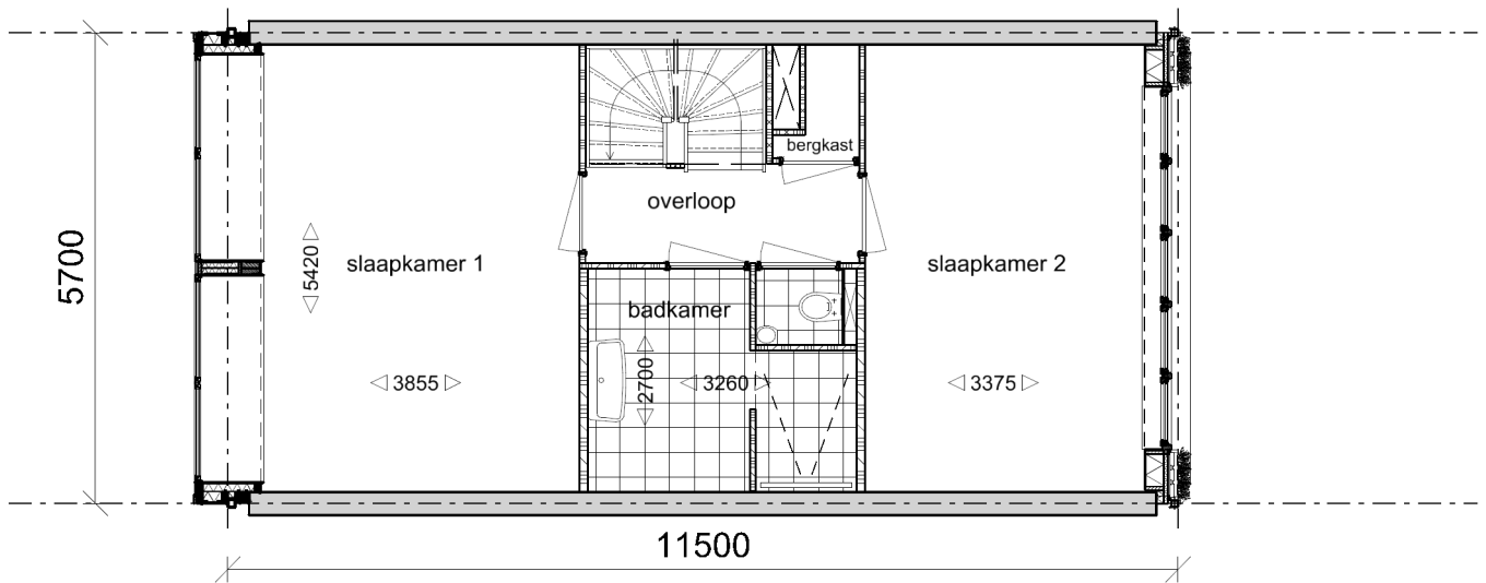
Verdieping 1
