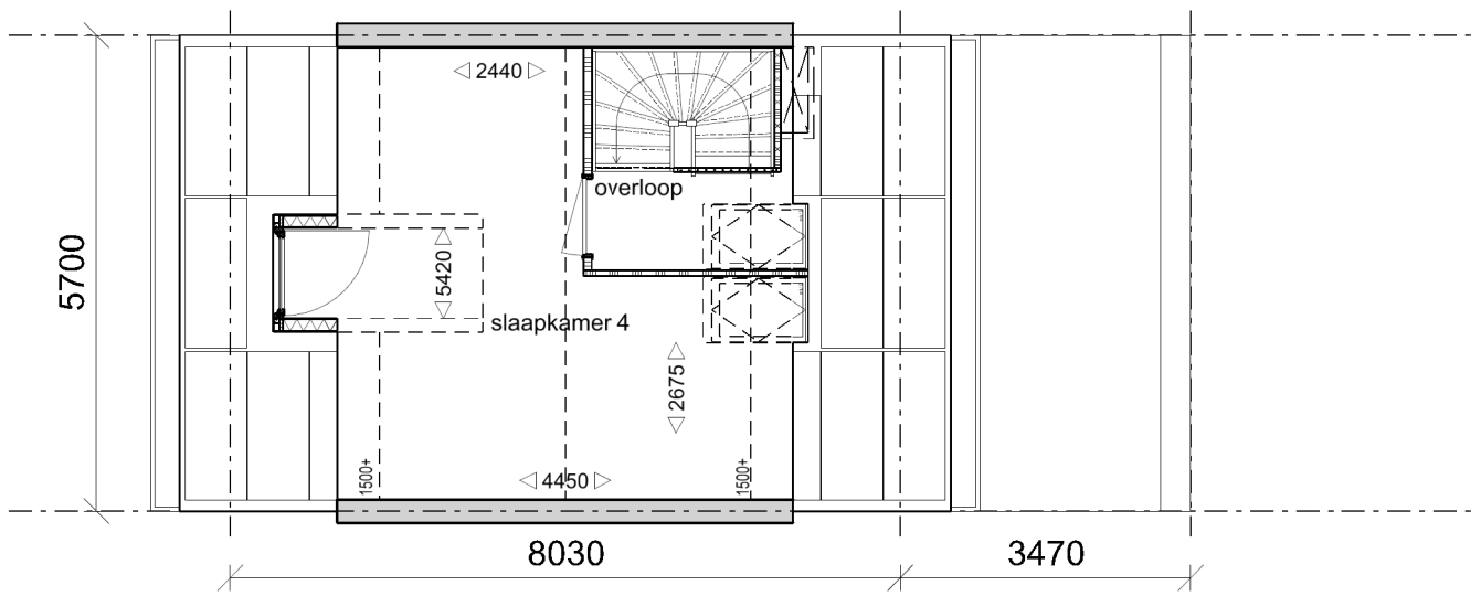
Verdieping 3
