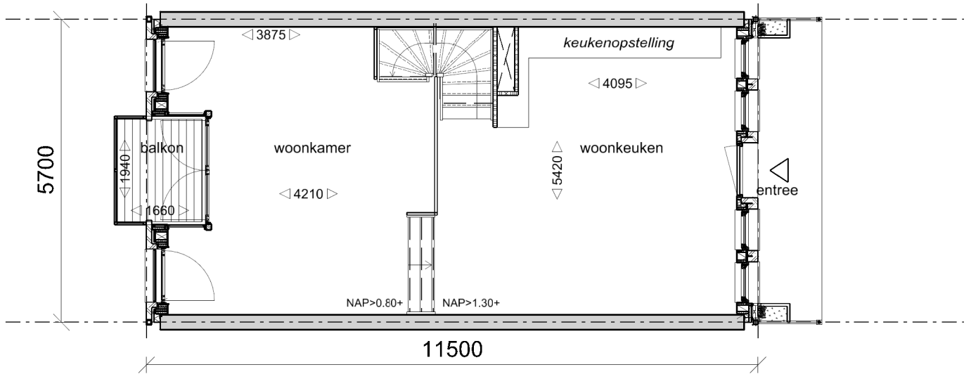
Begane grond
