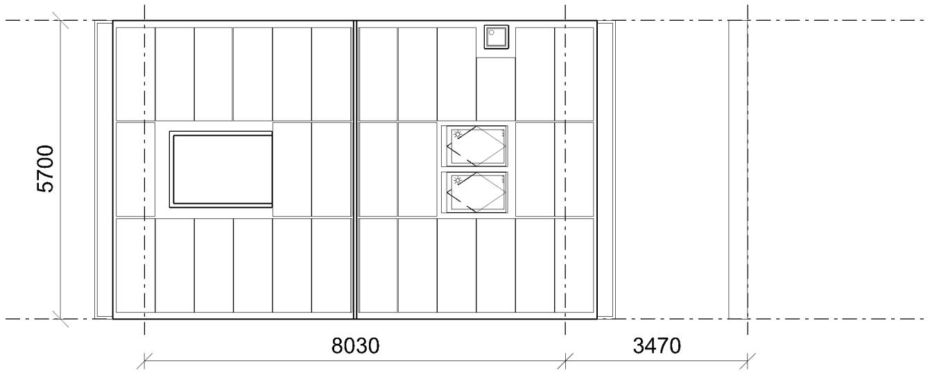
Dakaanzicht
