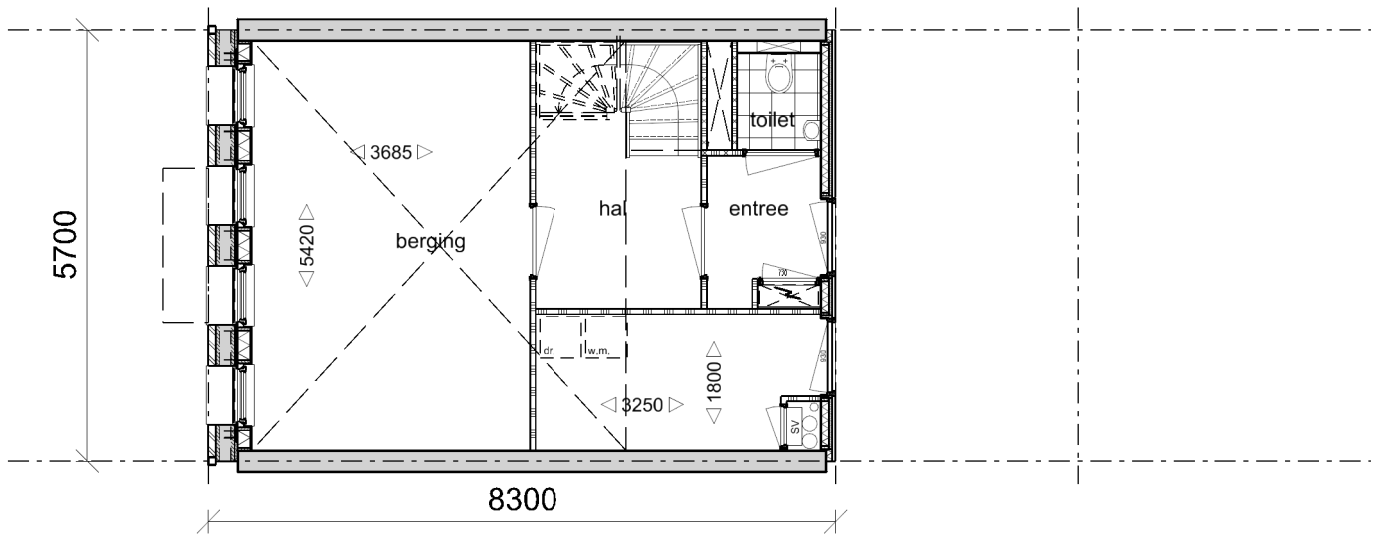
Souterrain
