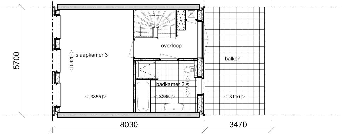
Verdieping 2
