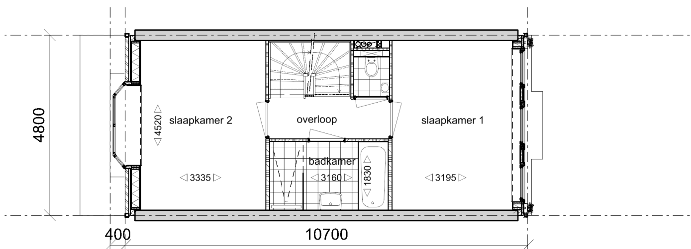
Verdieping 1
