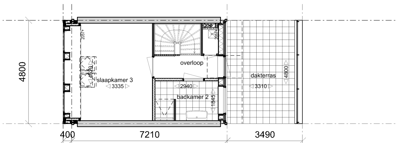
Verdieping 2
