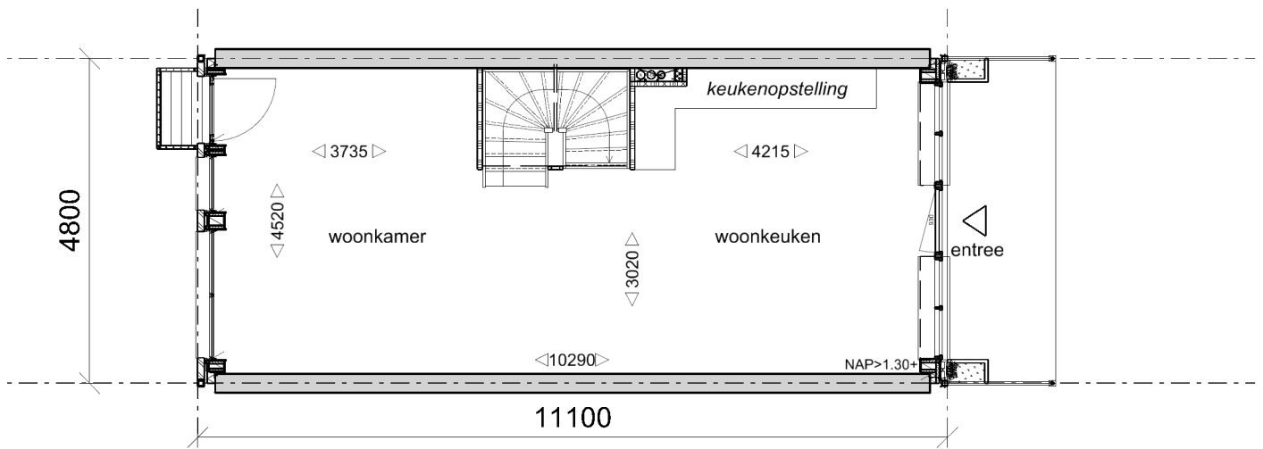
Begane grond
