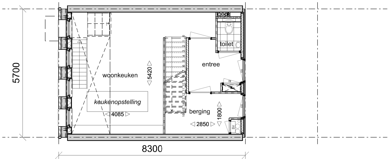
Souterrain
