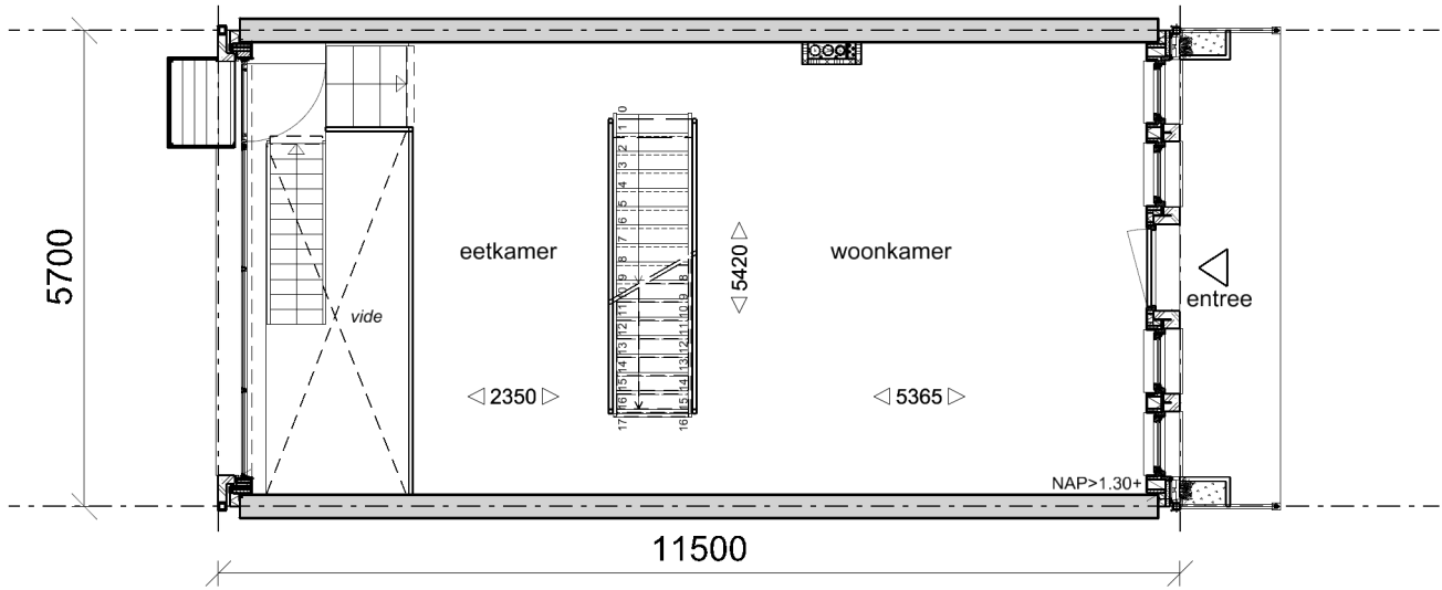
Begane grond
