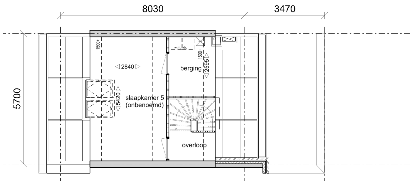
Verdieping 3
