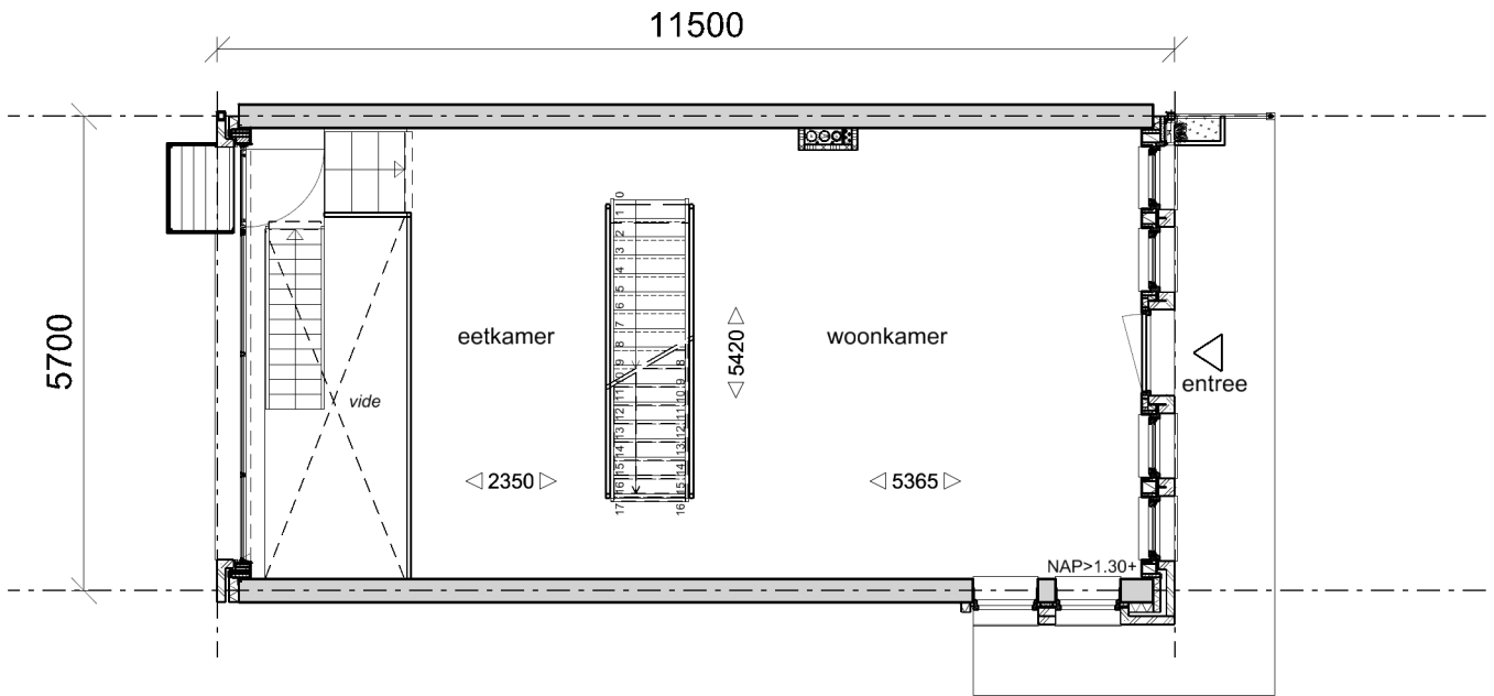
Begane grond
