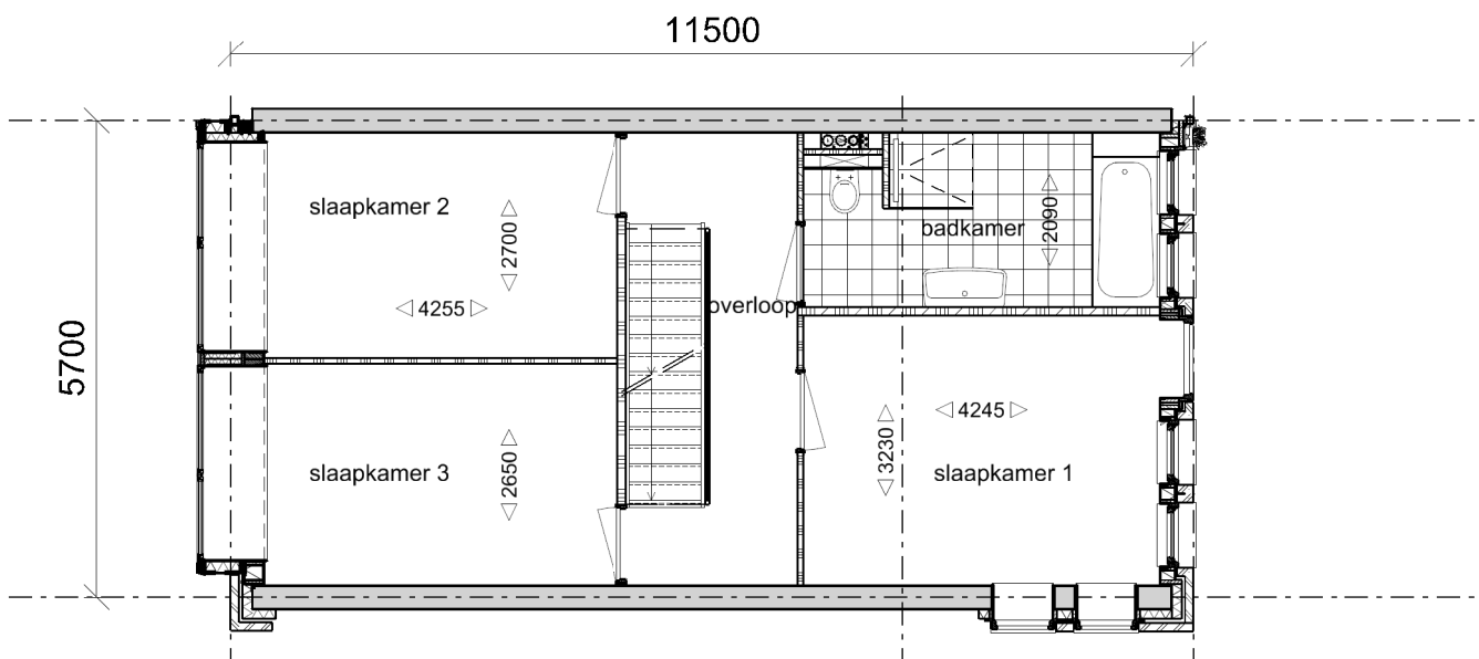
Verdieping 1
