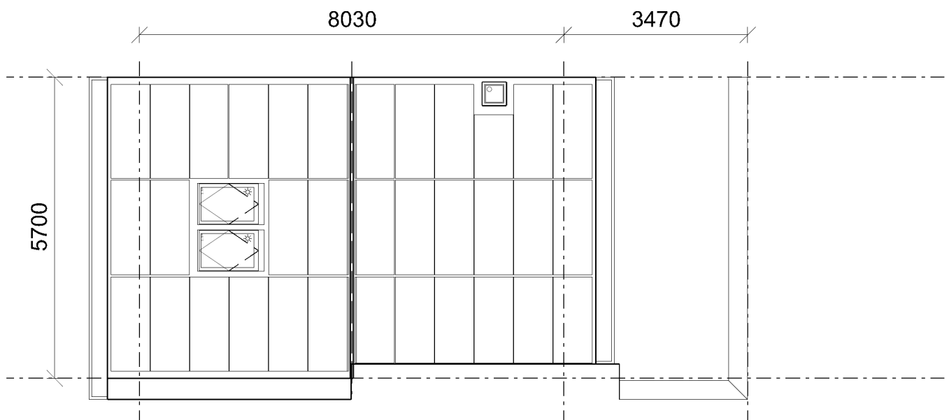
Dakaanzicht
