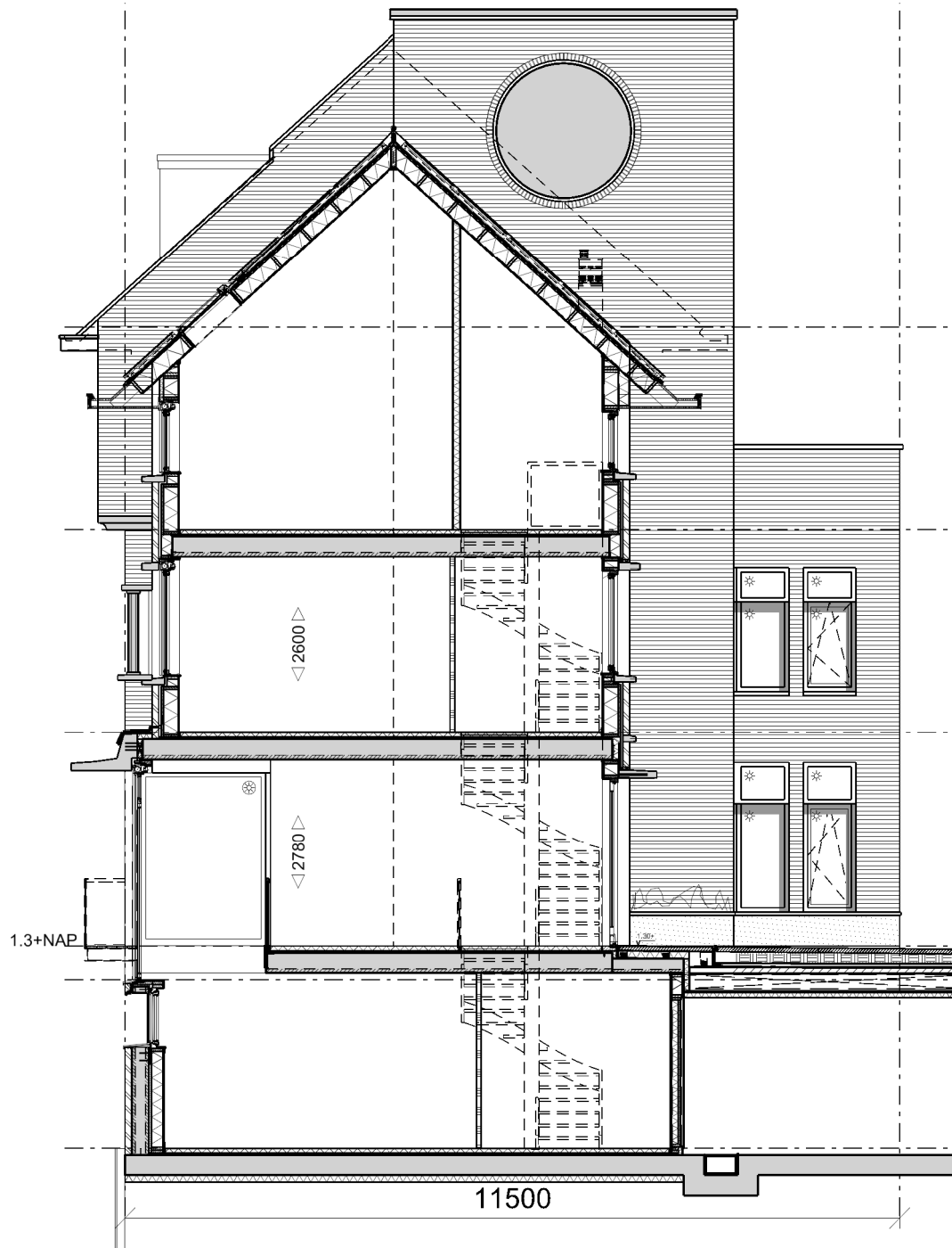
Zijgevel
