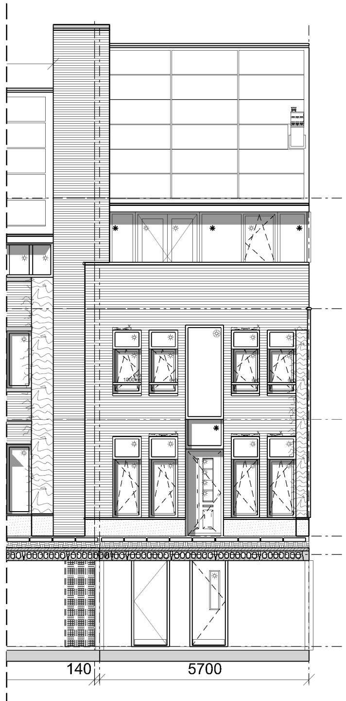
Gevel Straatzijde
