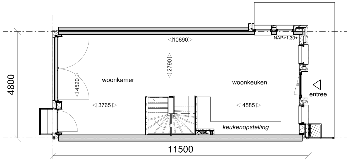
Begane grond
