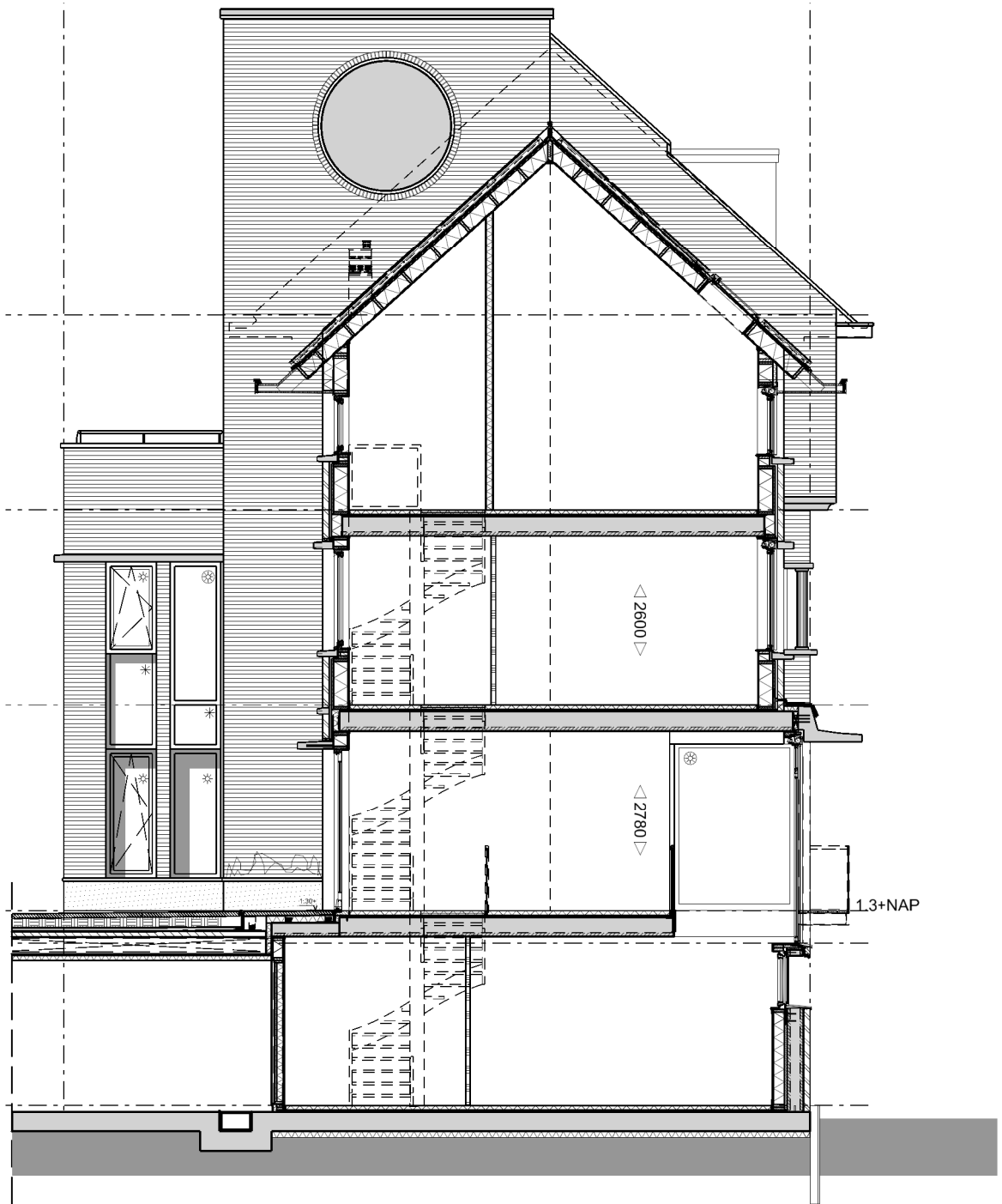
Zijgevel Plein
