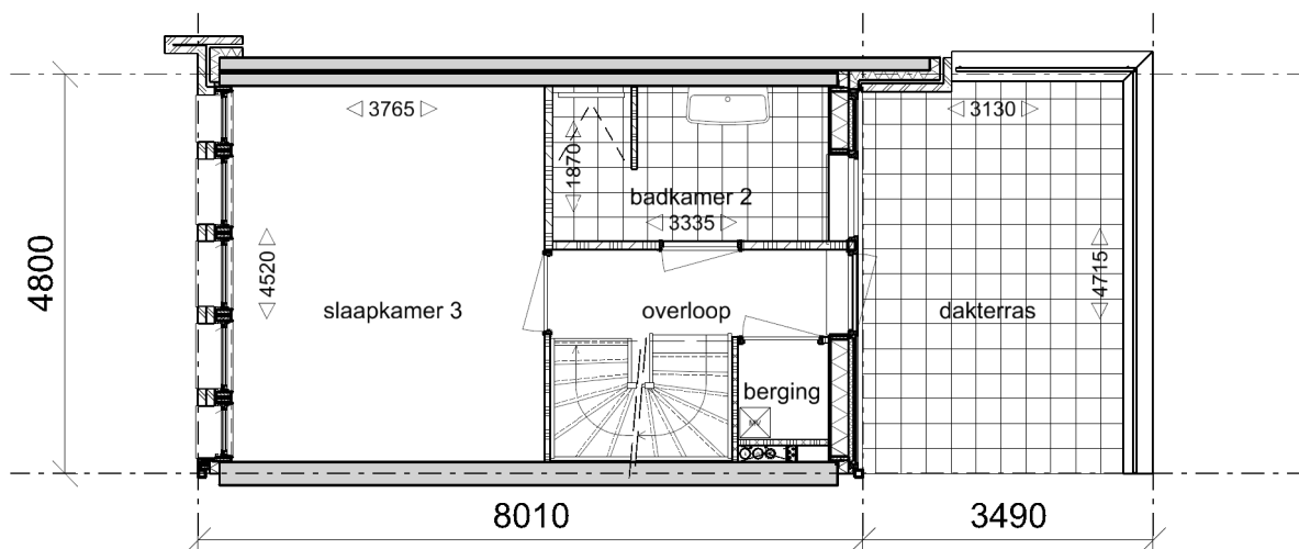
Verdieping 2
