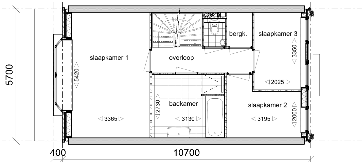
Verdieping 1
