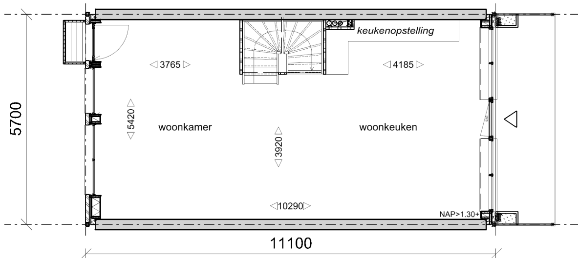
Begane grond
