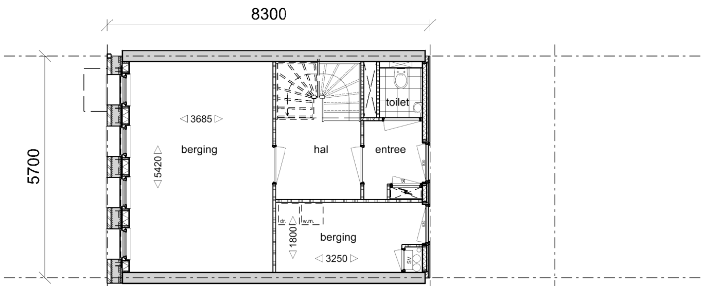
Souterrain
