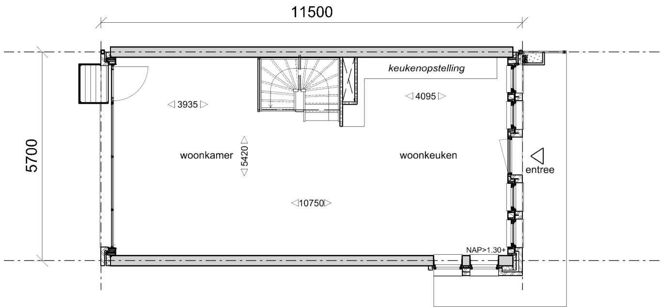
Begane grond
