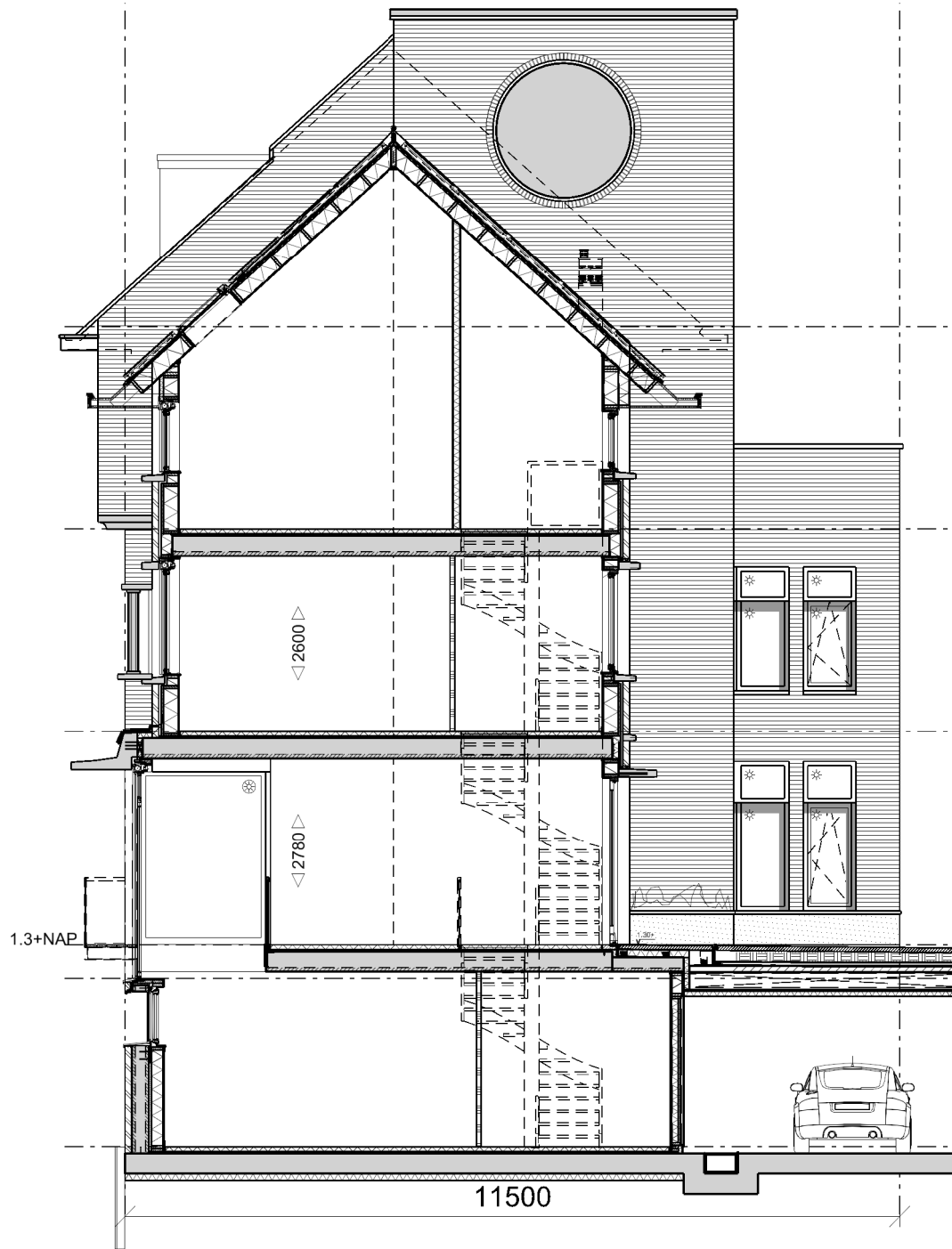
Zijgevel
